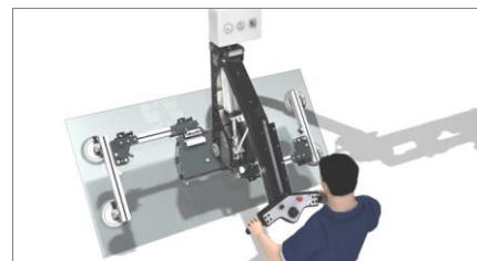
Mocowanie produktu 02
